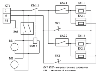
Рис.3. Схема электрическая ТЗС-508
