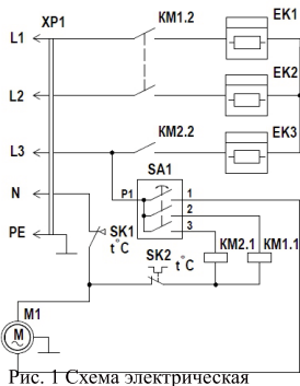
Рис. 1 Схема электрическая
